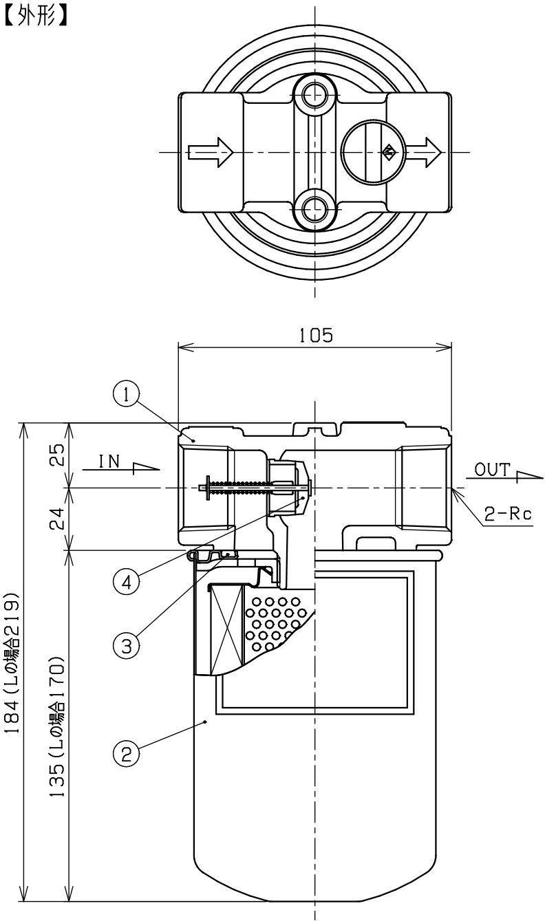
【寸法表】
